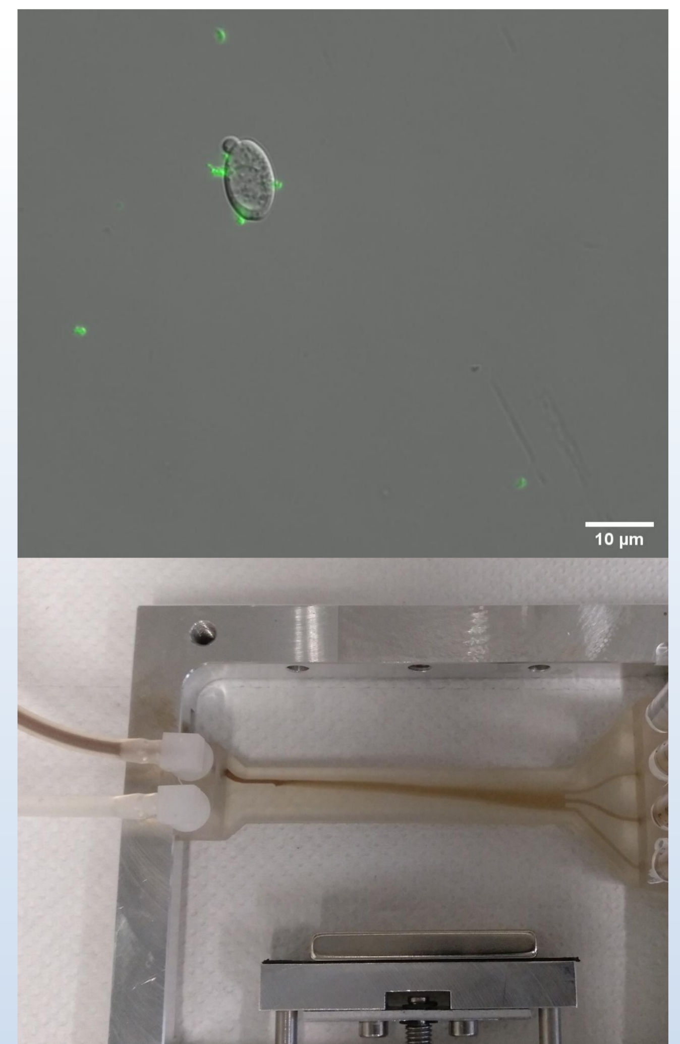
Oben: Fluoreszenzmarkierte Hefezellen mit Magnetischen Nanopartikeln. Unten: Set-up des Trennprozesses.
