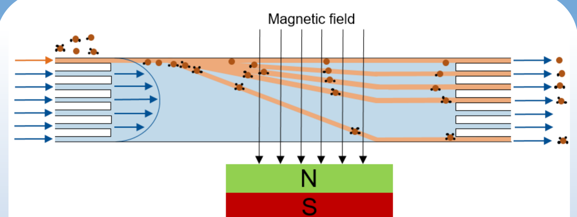
Prinzip der magnetischen Fraktionierung von Hefezellen durch einen millifluidischen Chip.
